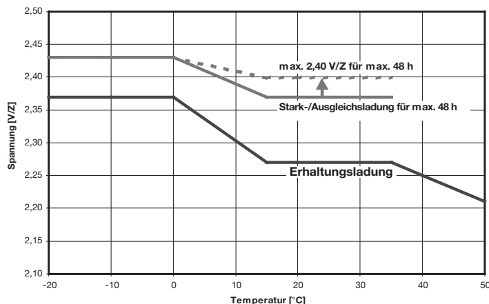
Bild 3: A 400/FT, PowerCycle; Ladespannung über der Temperatur
