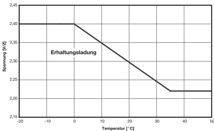
Bild 2: Marathon M/M-FT, Sprinter P/XP, Sprinter S; Ladespannung über der Temperatur
